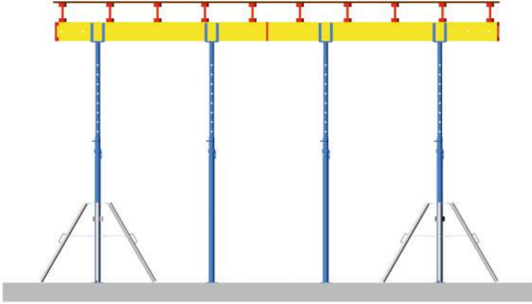
TAŞIMA KAPASİTESİ TABLOSU 'KG' EMNİYET KATSAYISI : 1,65
