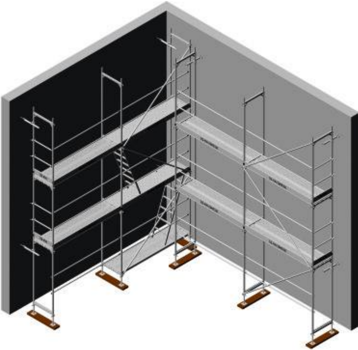
İç köşe iskele kurulum görünümü. Internal corner scaffold assembly view.
