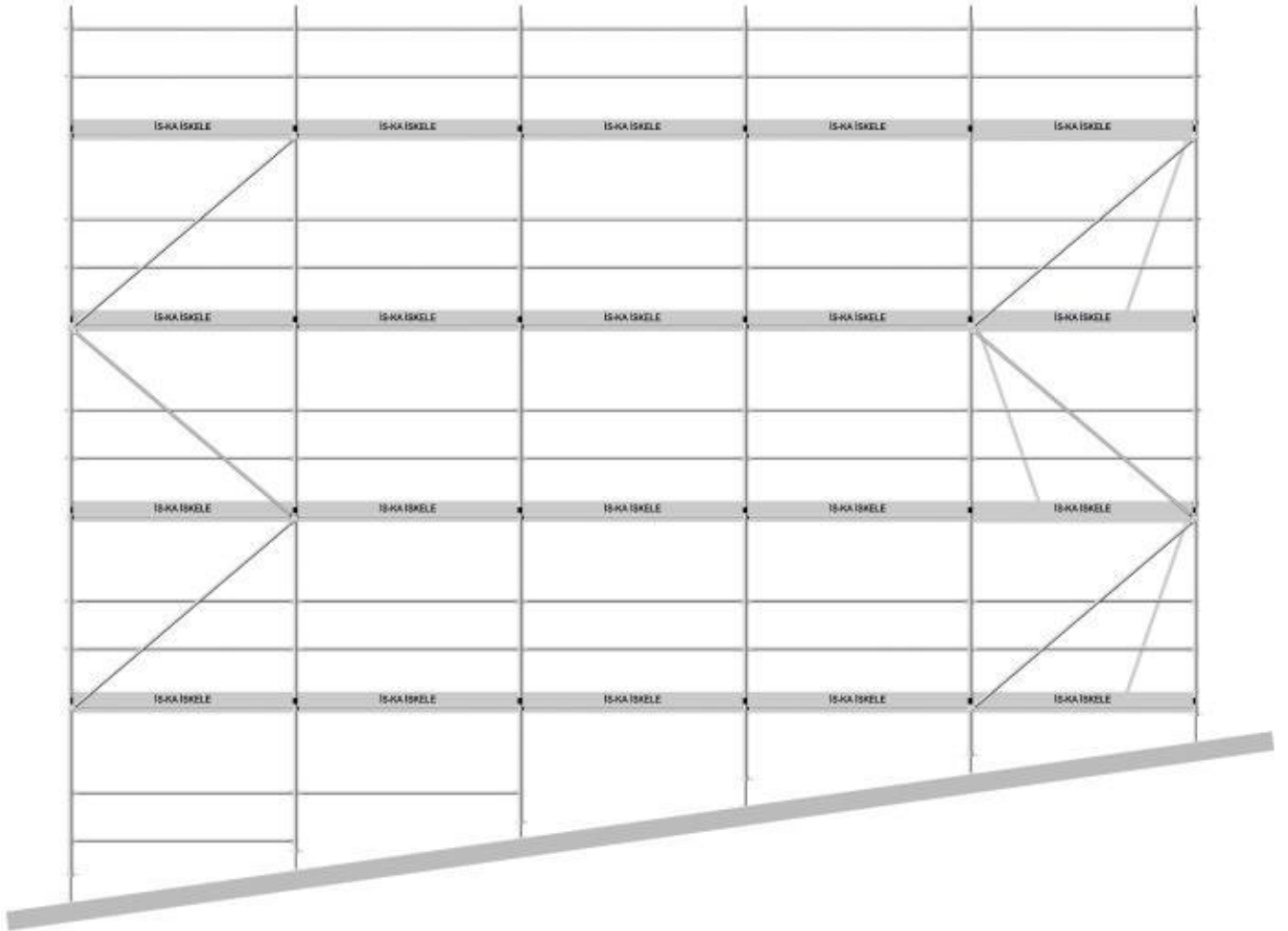
Eğimli cephelerde iskele görünüşü. Scaffolding appearance on sloping facades.
